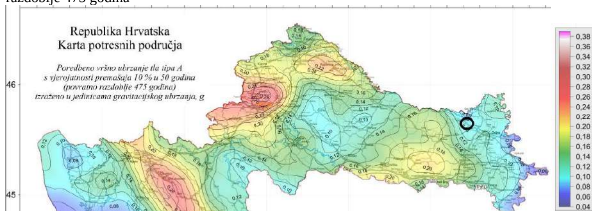
Slika 7: Jači potresi u Hrvatskoj od 1973.-2013.godine
