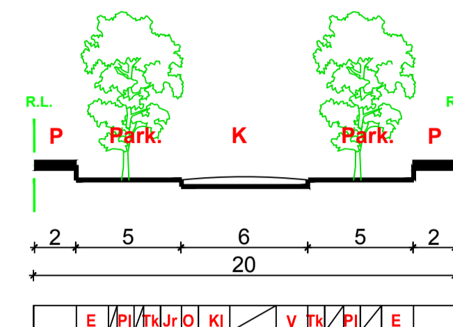
PRESJEK A-A
